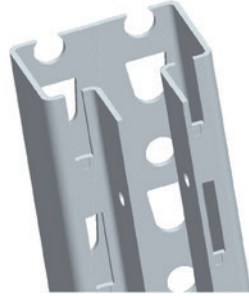
Schlitzung Slots
