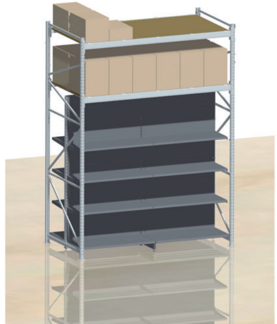
Integration Doppelreihe Integration double row
