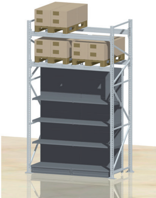
Palettenlängslagerung mit Integrierung Longitudinal storage of pallets with Integration
