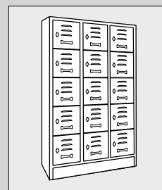
Fächersäule 15 Türen Fachmaß: 26 x 29 cm Breite: 105 cm Best.Nr. S15SM0101
