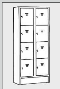
Fächersäule 8 Türen Fachmaß: 26 x 37 cm Breite: 70 cm Best.Nr. S08SM0101
