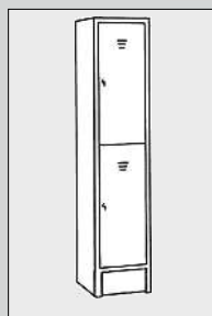
Schrank 2 Fächer Fachmaß: 26 x 76 cm Breite: 35 cm Best.Nr. 272SM0101
