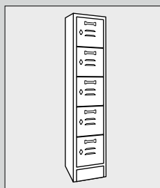
Fächersäule 5 Türen Fachmaß: 26 x 29 cm Breite: 35 cm Best.Nr. S05SM0101
