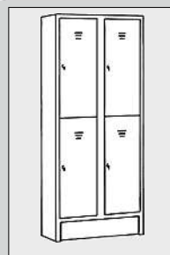
Schrank 4 Fächer Fachmaß: 26 x 76 cm Breite: 70 cm Best.Nr. 274SM0101
